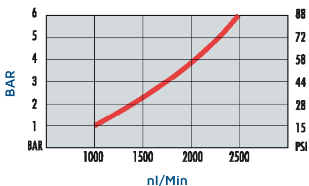
Průtok stlačeného vzduchu
